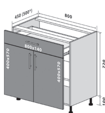
31 Низ 80-82 (1+2) Стандарт 31 Низ 80-82 (1+2) Люкс* 31 Bottom 80-82 (1+2) Standart 31 Bottom 80-82 (1+2) Luxe*
