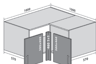
83 Верх 100-100 Люкс 83 Top 100-100 Luxe
