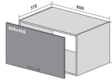
78 Верх 80-46 Стандарт 78 Верх 80-46 Люкс 78 Top 80-46 Standart 78 Top 80-46 Luxe
