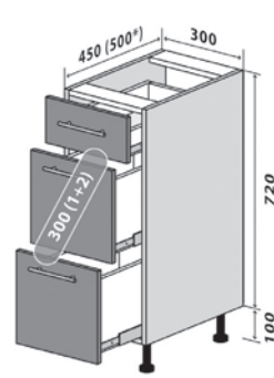
8 Низ 30-82 (1+2) Стандарт 8 Низ 30-82 (1+2) Люкс* 8 Bottom 30-82 (1+2) Standart 8 Bottom 30-82 (1+2) Luxe*
