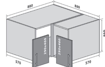
82 Верх 88-88 Стандарт 82 Top 88-88 Standart
