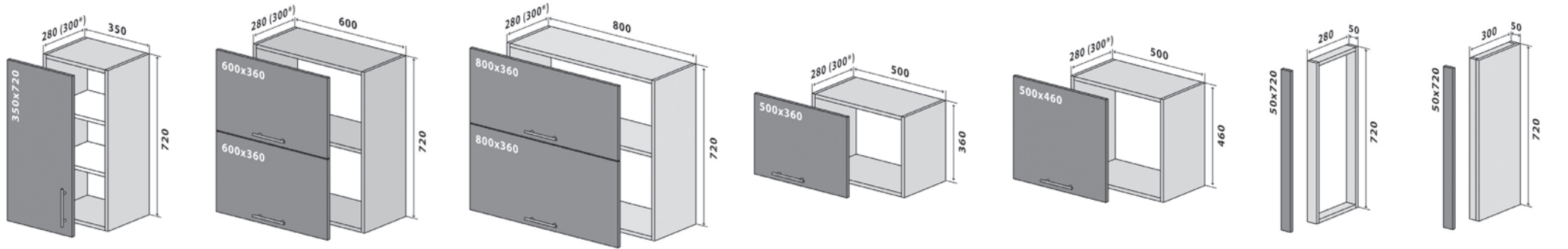
19 Верх 35-72 Стандарт 19 Верх 35-72 Люкс*
