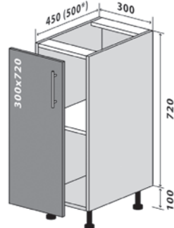
2 Низ 30-82 Стандарт 2 Низ 30-82 Люкс* 2 Bottom 30-82 Standart 2 Bottom 30-82 Luxe*
