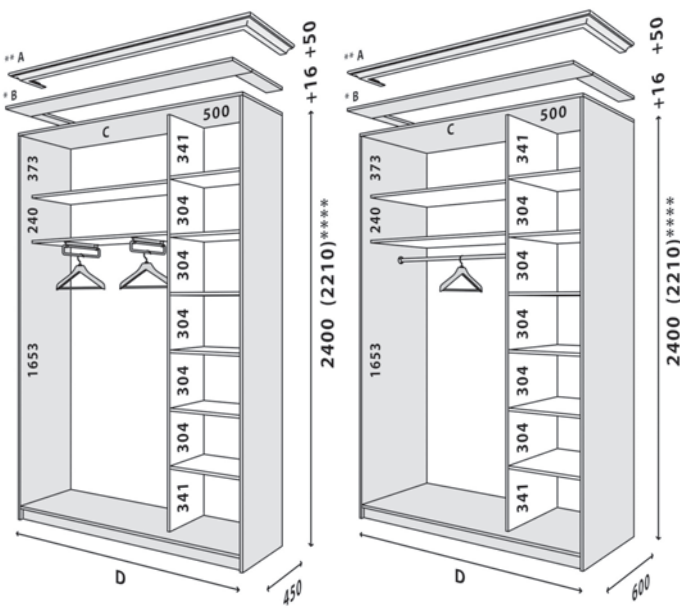
Схема шафи-купе на ширину 1600, 1700 Sliding wardrobe scheme for a width of 1600, 1700
