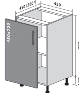
4 Низ 45-82 Стандарт 4 Низ 45-82 Люкс* 4 Bottom 45-82 Standart 4 Bottom 45-82 Luxe*
