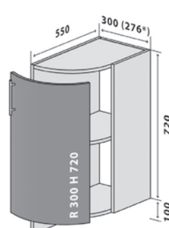
№17R Низ закінчення Стандарт №17R Низ закінчення Люкс* тільки кухні серії «МоДа», «Flat», «Margo», «Colour-mix» №17R Bottom end Standart №17R Bottom end Luxe* kitchen series only «MoDa», «Flat», «Margo», «Colour-mix»
