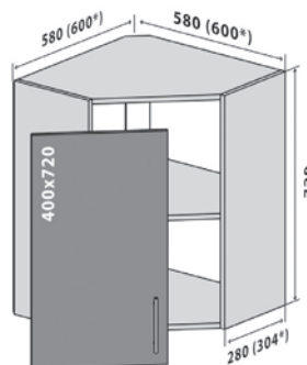
14 Верх 58-58 Стандарт 14 Верх 60-60 Люкс* (можлива вітрина)
