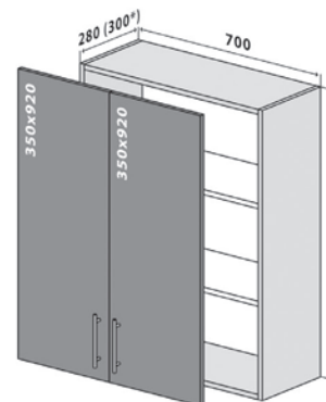
88 Верх 70-92 Стандарт 88 Верх 70-92 Люкс* 88 Top 70-92 Standart 88 Top 70-92 Luxe*
