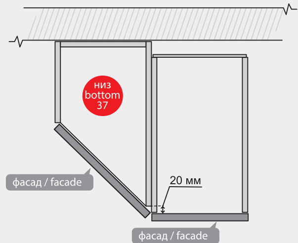
Схема монтажу модуля низ 37. Installation diagram for bottom module 37.
