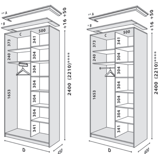
Схема шафи на ширину 1100, 1200 Sliding wardrobe scheme for a width of 1100, 1200 ширина width A B C D фасад front 1100 1201 1101 552 1101 550 1200 1301 1201 652 1201 590
