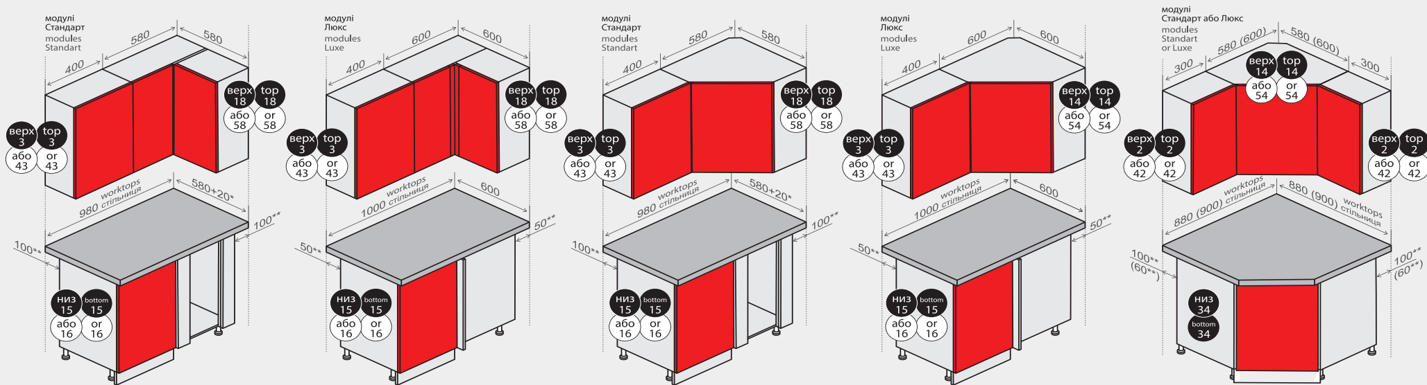
Схеми варіантів кутового з'єднання кухонних модулів. | Schemes of corner connection of kitchen modules.
