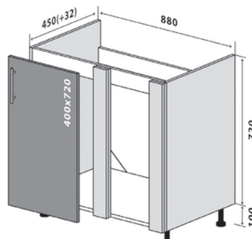
15 Низ Мийка УНІ 88-82 Стандарт 15 Bottom Sink UNI 88-82 Standart
