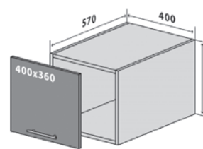
65 Verx 40-36 Стандарт 65 Verx 40-36 Люкс
