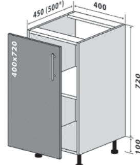
3 Низ 40-82 Стандарт 3 Низ 40-82 Люкс* 3 Bottom 40-82 Standart 3 Bottom 40-82 Luxe*
