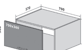
67 Verx 70-36 Стандарт 67 Verx 70-36 Люкс
