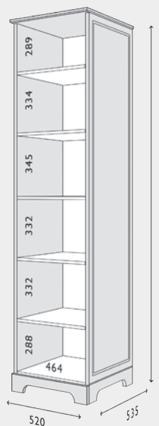
Схема пеналу без фасаду Модуль М-1 Мадрид Case layout without front Module M-1 Madrid
