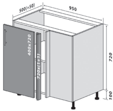
16 Низ УНІ 95-82 Люкс 16 Bottom UNI 95-82 Luxe
