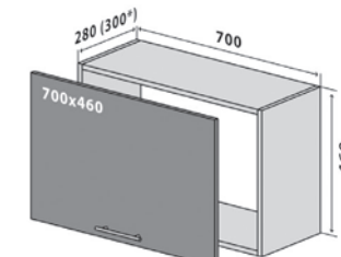
85 Верх 70-46 Стандарт 85 Верх 70-46 Люкс* 85 Top 70-46 Standart 85 Top 70-46 Luxe*
