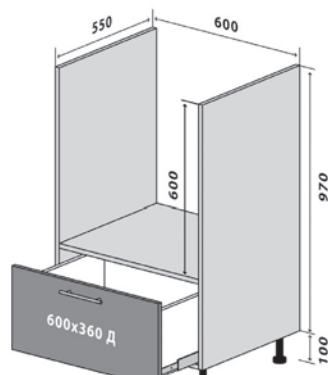
32 Низ 60-107 (1) Стандарт 32 Низ 60-107 (1) Люкс 32 Bottom 60-107 (1) Standart 32 Bottom 60-107 (1) Luxe
