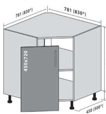
34 Низ на кут 78-78 Стандарт 34 Низ на кут 83-83 Люкс* 34 Bottom corner 78-78 Standart 34 Bottom corner 83-83 Luxe*
