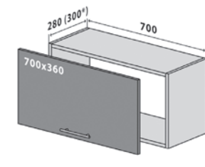
84 Верх 70-36 Стандарт 84 Верх 70-36 Люкс* 84 Top 70-36 Standart 84 Top 70-36 Luxe*
