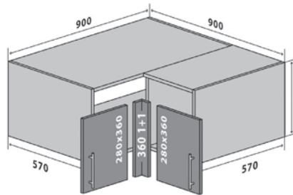
80 Верх 90-90 Люкс 80 Top 90-90 Luxe
