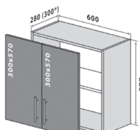
53 Verx 60-57,7 Стандарт 53 Verx 60-57,7 Люкс*
