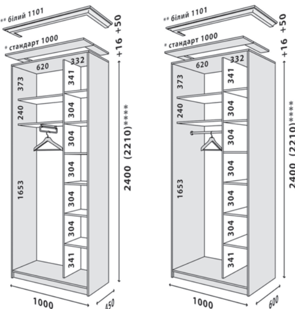
Схема шафи-купе на ширину 1000***, фасад 500 ***не може комплектуватися шухлядами Sliding wardrobe scheme for a width of 1000, with a 500 front ***cannot be equipped with drawers
