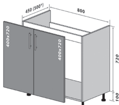
14 Низ Мийка 80-82 Стандарт 14 Низ Мийка 80-82 Люкс* 14 Bottom Sink 80-82 Standart 14 Bottom Sink 80-82 Luxe*
