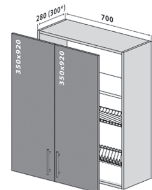
89 Верх 70-92 Стандарт 89 Верх 70-92 Люкс* сушка Стандарт в комплекті сушка Люкс* не входить в комплект 89 Top 70-92 Standart 89 Top 70-92 Luxe* drying Standart* Included drying Luxe* is not included
