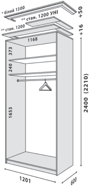
Схема шафи-купе на ширину 1200 УНІ, фасад 590 Sliding wardrobe scheme for a width of 1200 UNI, with a 590 front
