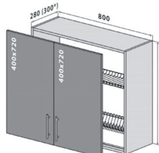
9 Верх 80-72 Стандарт 9 Верх 80-72 Люкс* сушка Стандарт в комплекті сушка Люкс* не входить в комплект (можлива вітрина)
