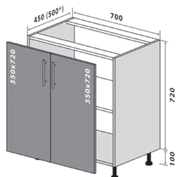
43 Низ 70-82 Стандарт 43 Низ 70-82 Люкс*
