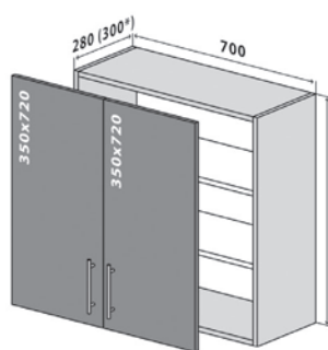
86 Верх 70-72 Стандарт 86 Верх 70-72 Люкс* 86 Top 70-72 Standart 86 Top 70-72 Luxe*
