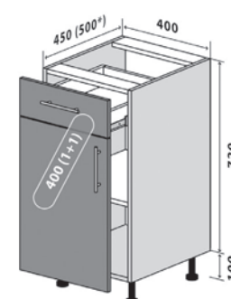
23 Низ 40-82 (1+1) Стандарт 23 Низ 40-82 (1+1) Люкс* 23 Bottom 40-82 (1+1) Standart 23 Bottom 40-82 (1+1) Luxe*
