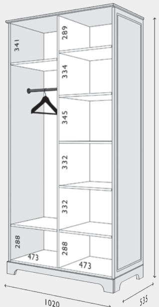
Схема шафи без фасаду Модуль М-2 Мадрид Wardrobe layout without front Module M-2 Madrid
