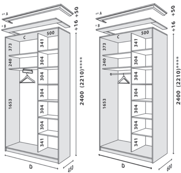
Схема шафи-купе на ширину 1300, 1400, 1500 Sliding wardrobe scheme for a width of 1300, 1400, 1500
