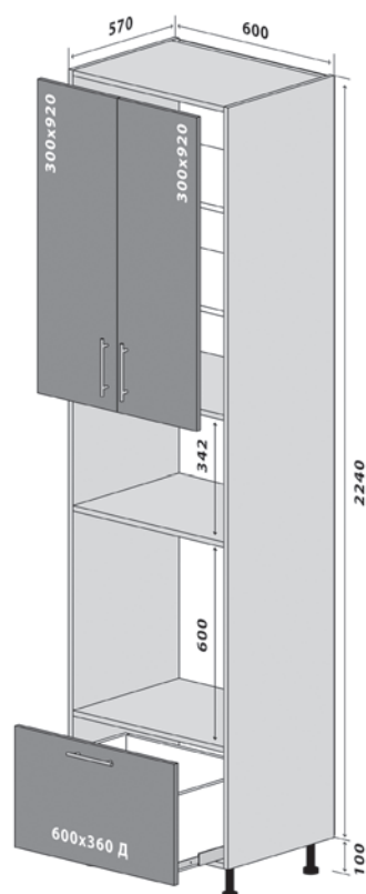
41 Низ Пенал 60-234 Стандарт 41 Низ Пенал 60-234 Люкс
