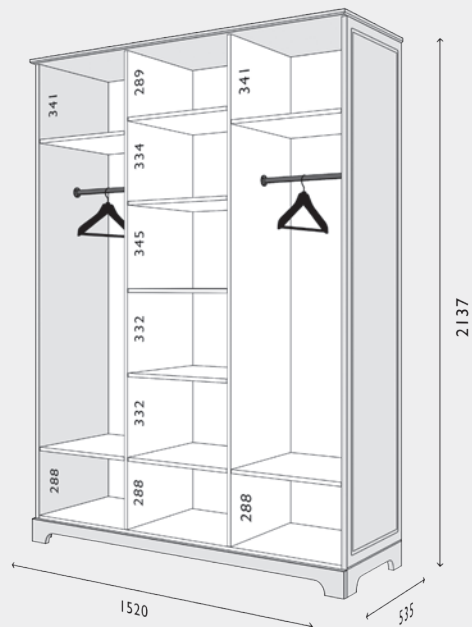
Схема шафи без фасаду Модуль М-3 Мадрид Wardrobe layout without front Module M-3 Madrid
