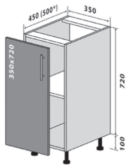
25 Низ 35-82 Стандарт 25 Низ 35-82 Люкс* 25 Bottom 35-82 Standart 25 Bottom 35-82 Luxe*
