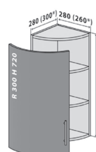
15R Верх Верх закінчення Стандарт 15R Верх Верх закінчення Люкс* збирайте як на ліву, так і на праву сторону тільки кухні серії «МоДа», «Flat», «Margo», «Colour-mix»
