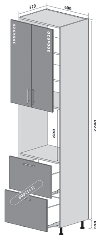
21 Низ Пенал 60-234 Стандарт 21 Низ Пенал 60-234 Люкс
