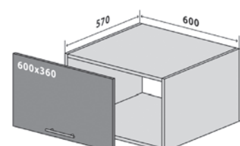
66 Verx пенал 60-36 Стандарт 66 Verx пенал 60-36 Люкс (можлива вітрина)
