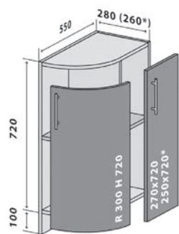
37R Низ закінчення 30-82 Стандарт 37R Низ закінчення 30-82 Люкс* тільки кухні серії «МоДа», «Flat», «Margo», «Colour-mix»
