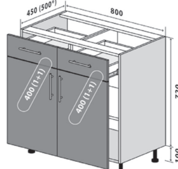
27 Низ 80-82 (2+2) Стандарт 27 Низ 80-82 (2+2) Люкс* 27 Bottom 80-82 (2+2) Standart 27 Bottom 80-82 (2+2) Luxe*
