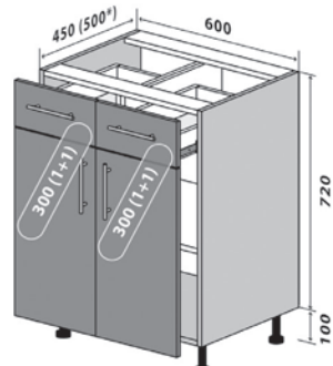
26 Низ 60-82 (2+2) Стандарт 26 Низ 60-82 (2+2) Люкс* 26 Bottom 60-82 (2+2) Standart 26 Bottom 60-82 (2+2) Luxe*
